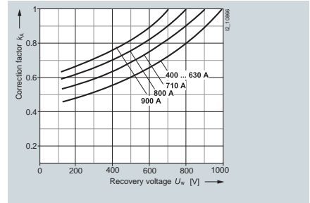
分断 I^2t 值修正系数
