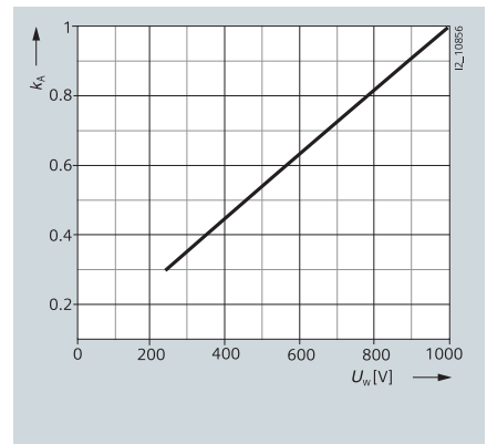
分断 I^2t 值修正系数
